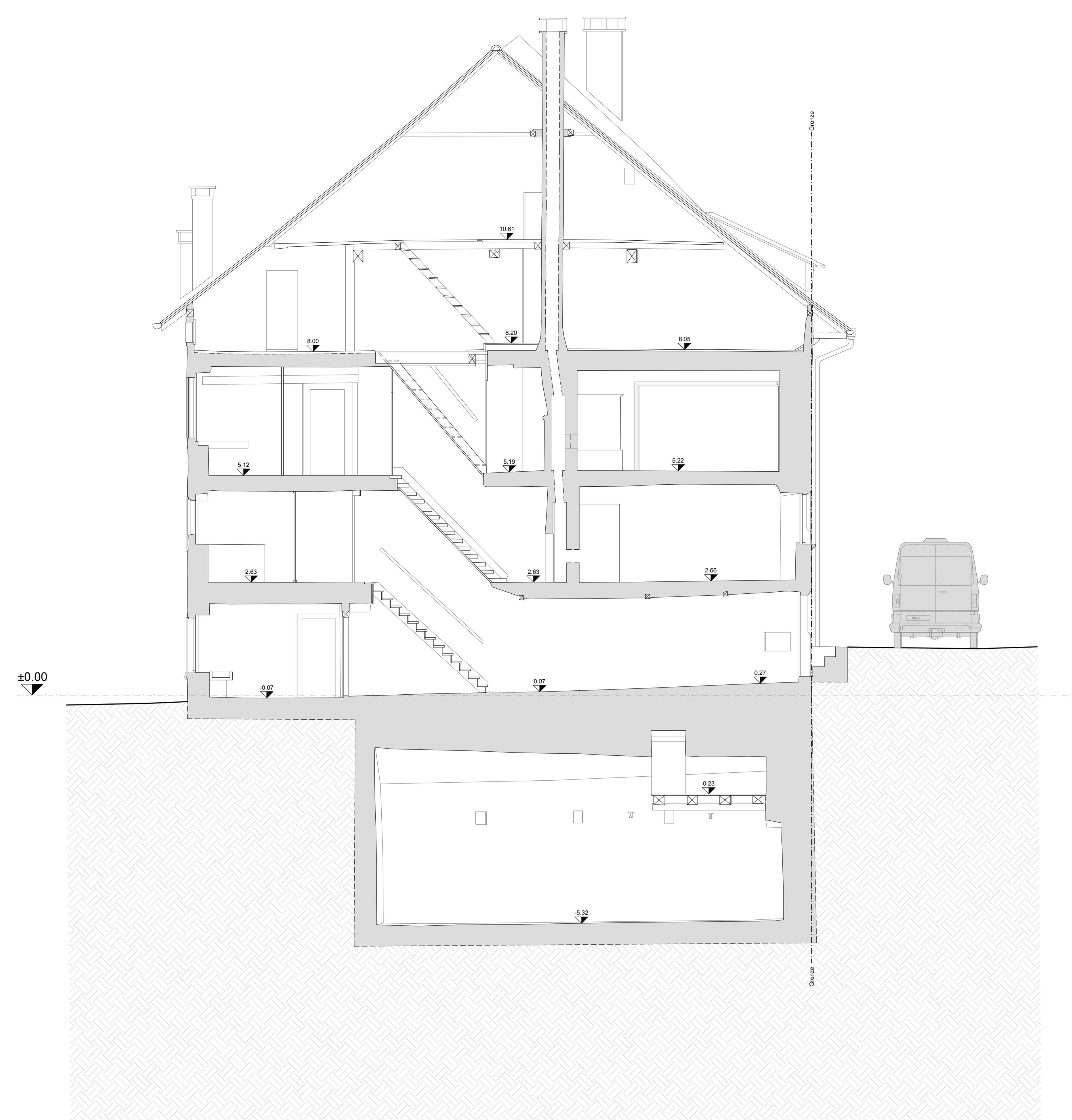
Schnitt F-F M 1:50
