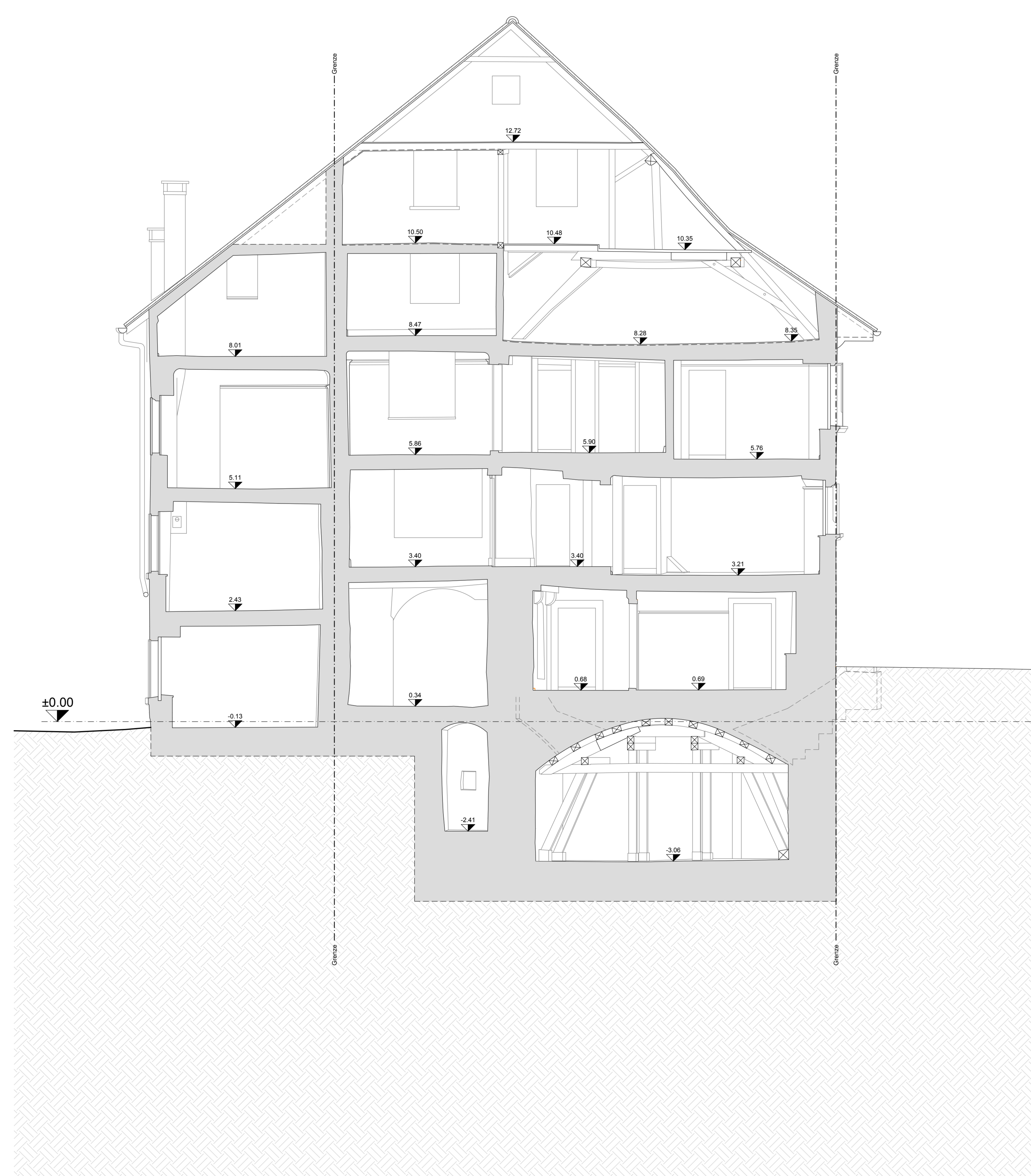
Schnitt G-G M 1:50
