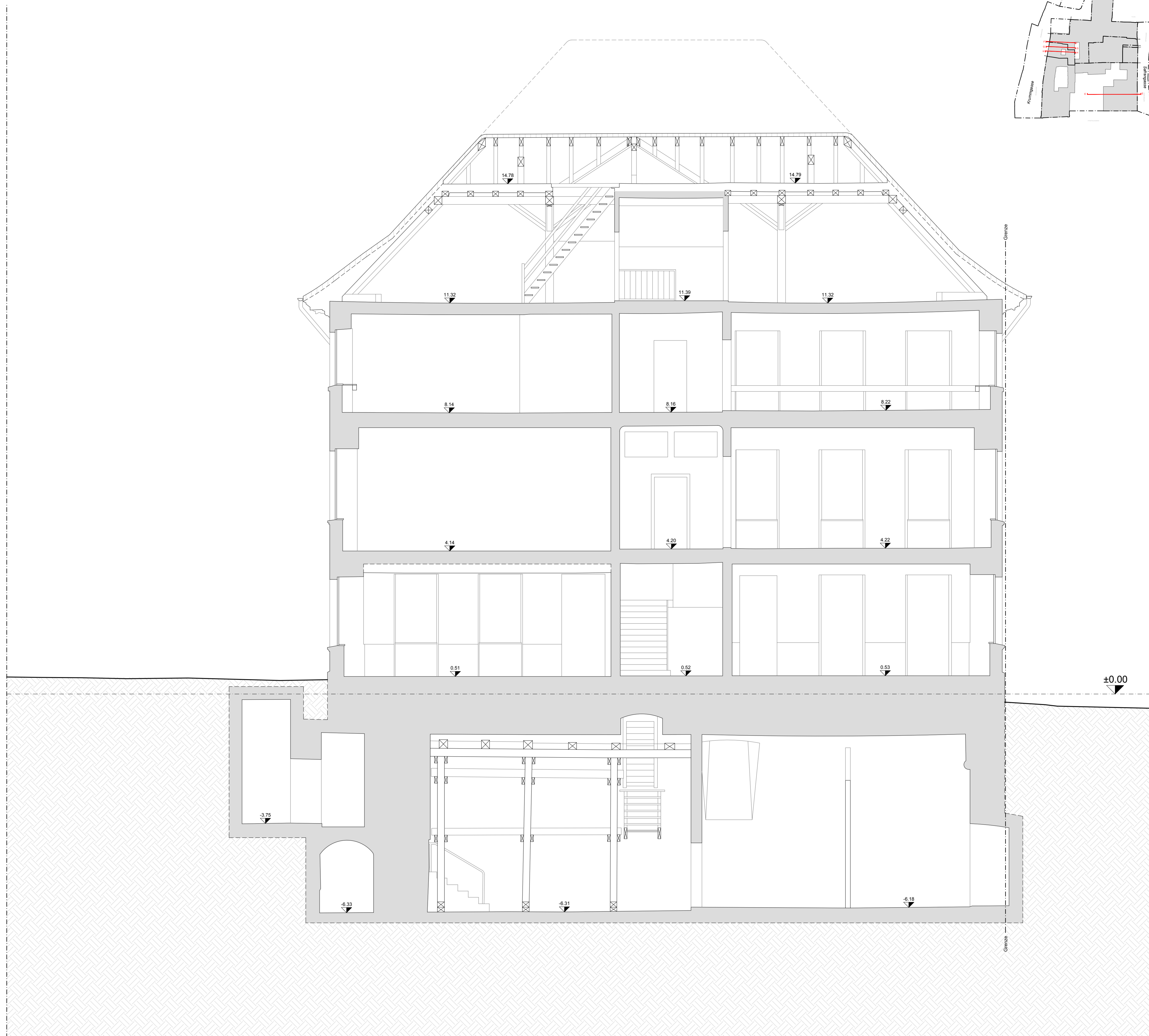
Schnitt E-E M 1:50
