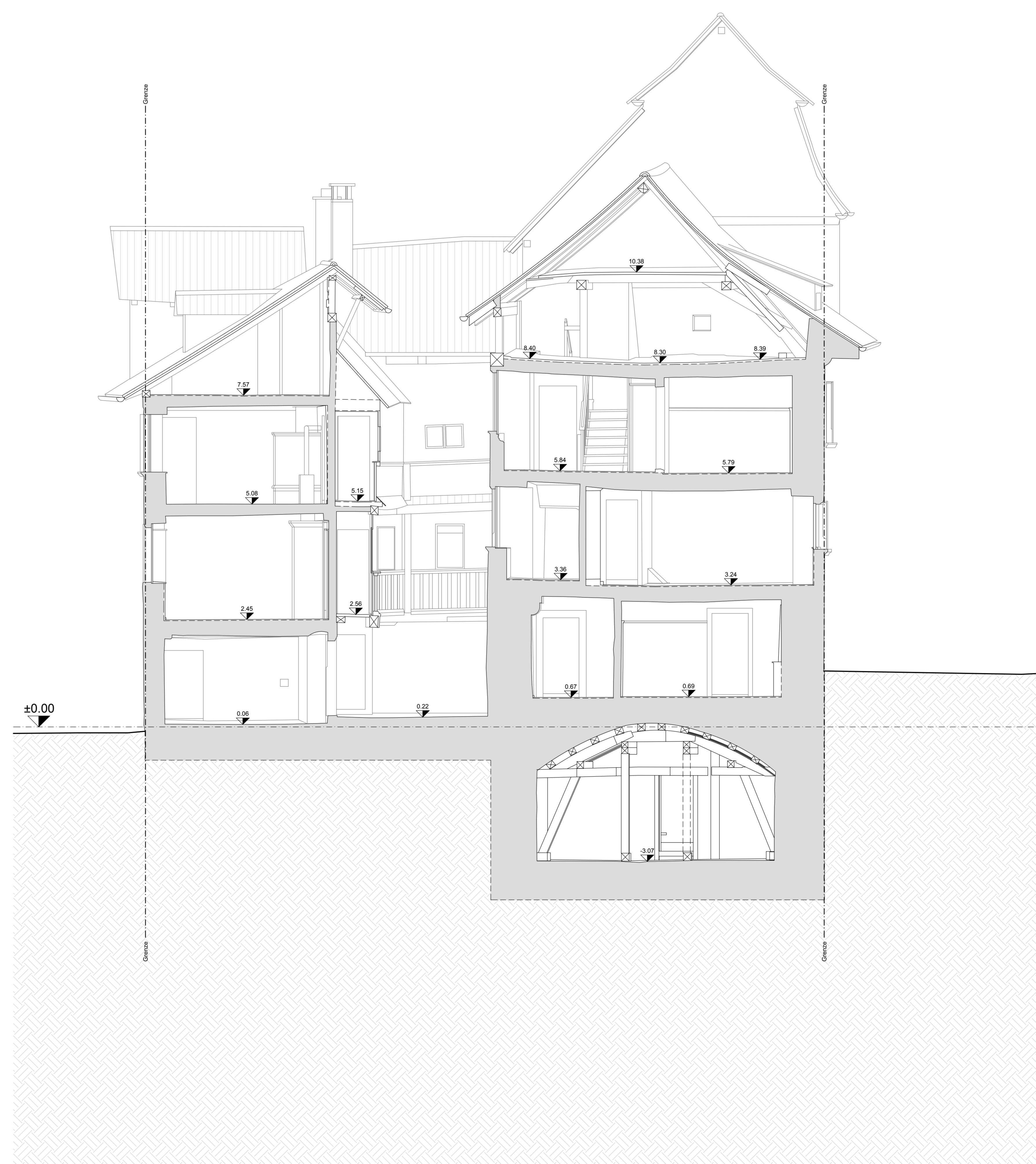
Schnitt H-H M 1:50
