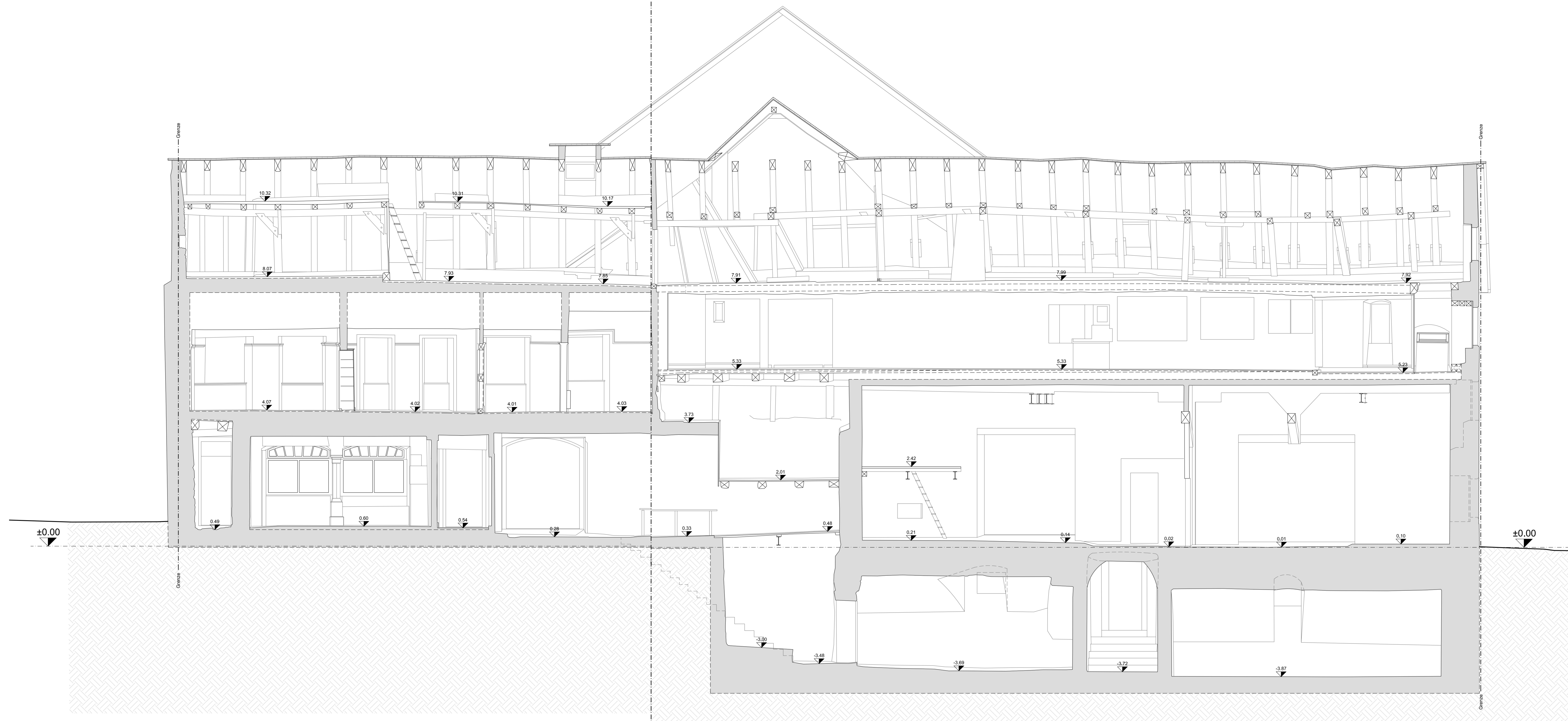
Schnitt A-A M 1:50
