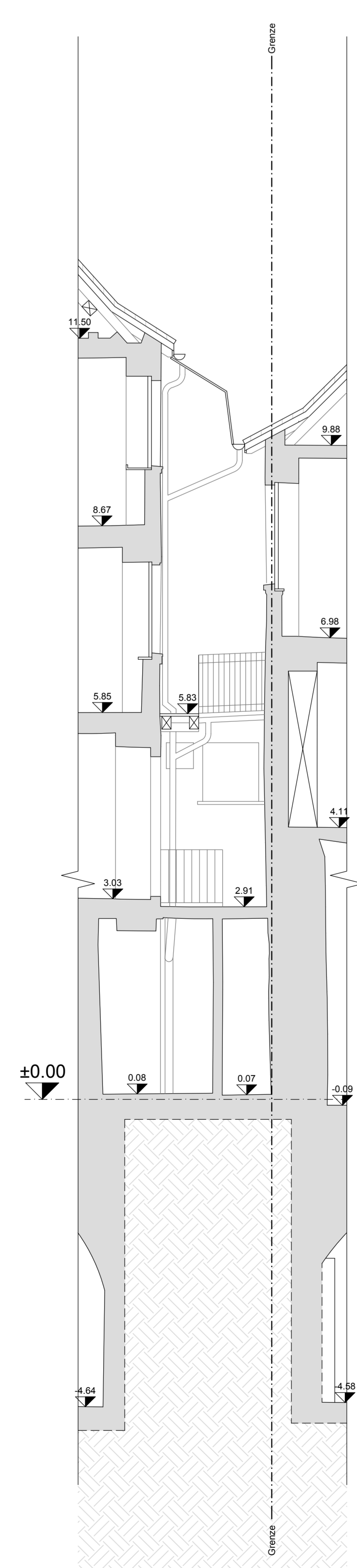
Schnitt C-C M 1:50
